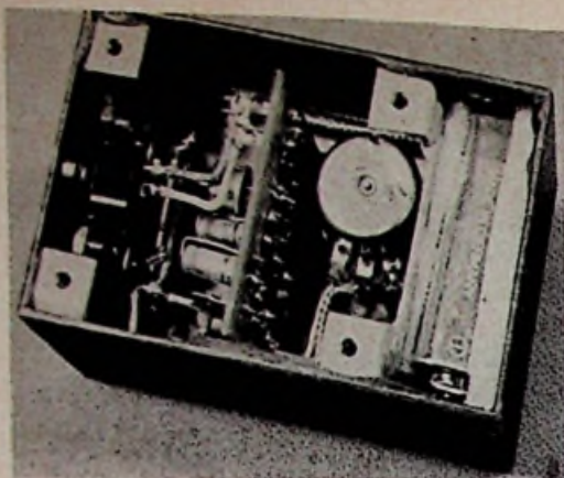
Afb. 7. Onderaanzicht van afgemonteerde meeluisterversterker.
